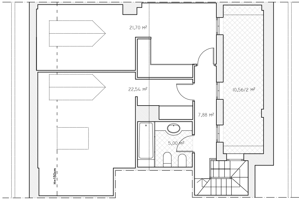
PLANTA 4ª SUP. ÚTIL 62,40 m²
